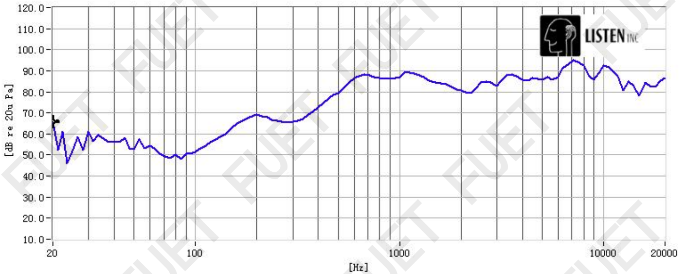
頻响曲线
