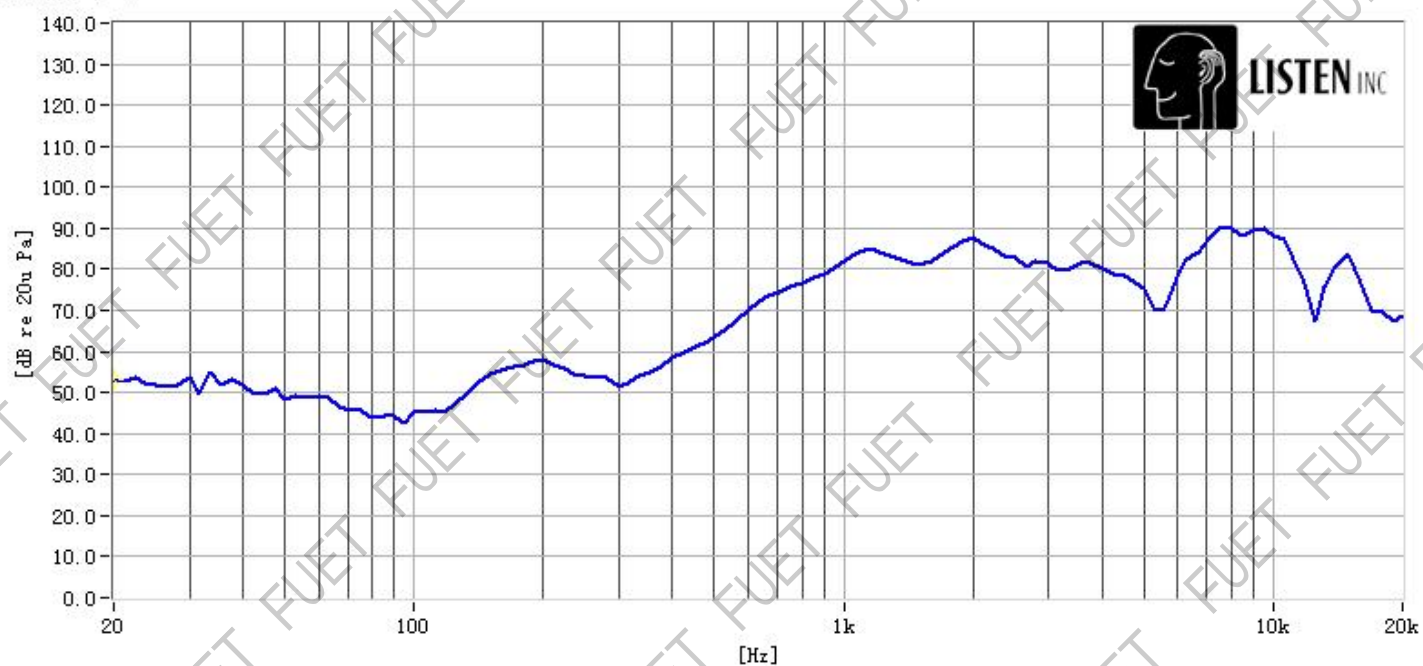
频响曲线
