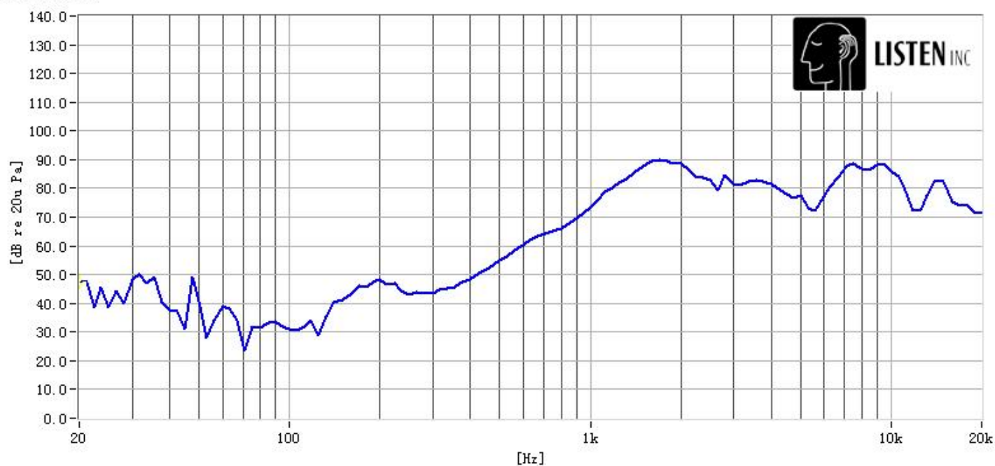
频响曲线
